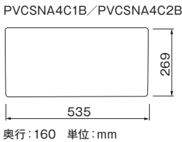
〈昇圧回路付接続箱 外形図〉
