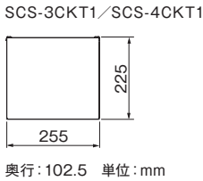
〈接続箱 外形図〉
