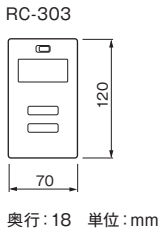
〈リモコン 外形図〉
