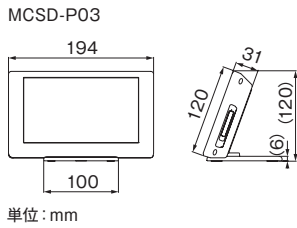
〈カラーモニター 外形図〉
