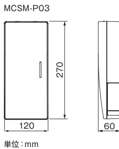
〈送信ユニット 外形図〉
