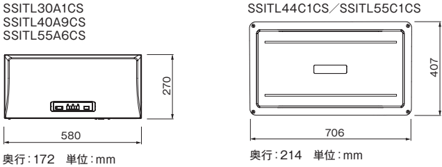
〈パワーコンディショナ 外形図〉
